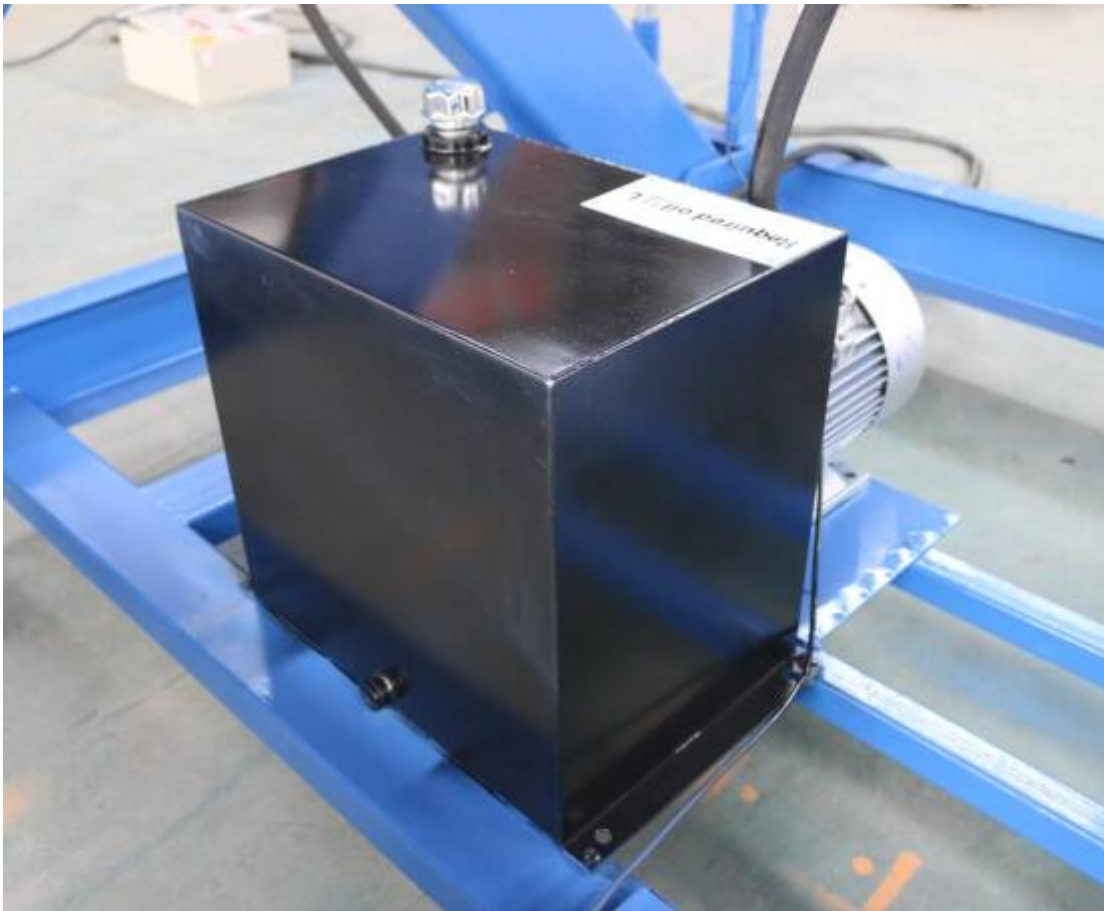
Tanque de aceite hidráulico
